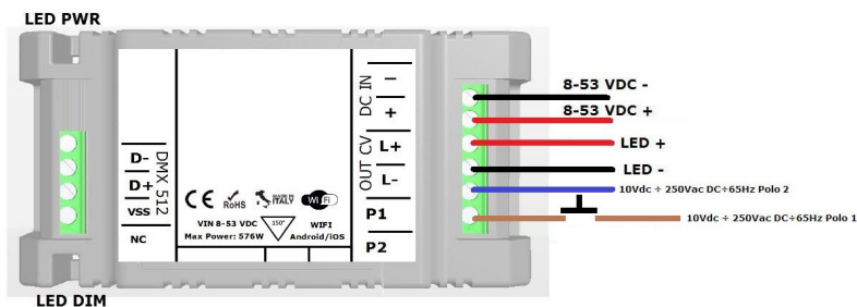
COLLEGAMENTO PULSANTE L458MA04T1A01 - FIGURA N. 2
