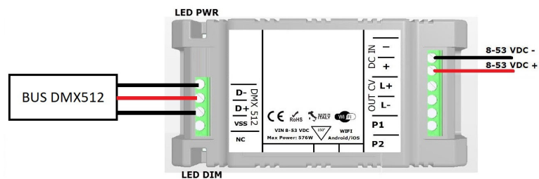
COLLEGAMENTO WIFI + DMX L458MA04T1A01 - FIGURA N. 5
