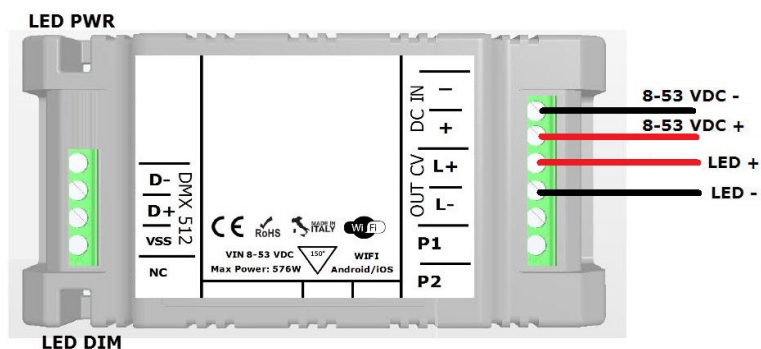
SCHEMA COLLEGAMENTO ALIMENTAZIONE E LED L458MA04T1A01 - FIGURA N. 1
