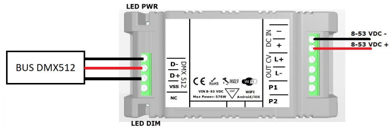
WIFI + DMX L458MA04T1A01 WIRING - FIGURA N. 5
