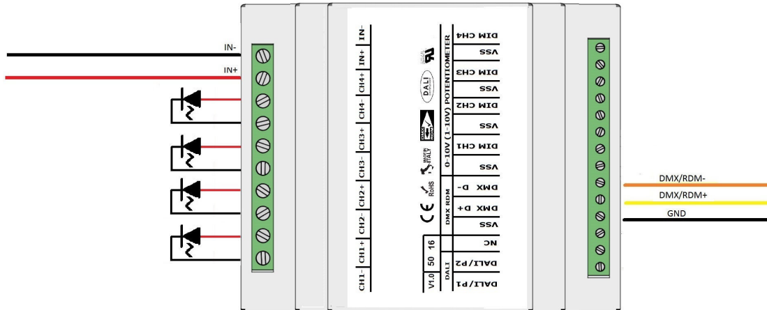
COLLEGAMENTO L405MA02C4A01 A BUS DMX512/RDM - FIGURA N. 4
